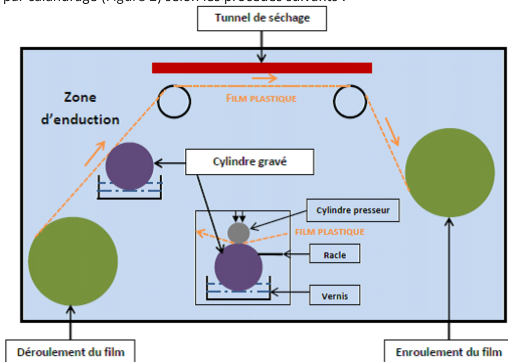
Figure 1 : Procédé d'enduction
